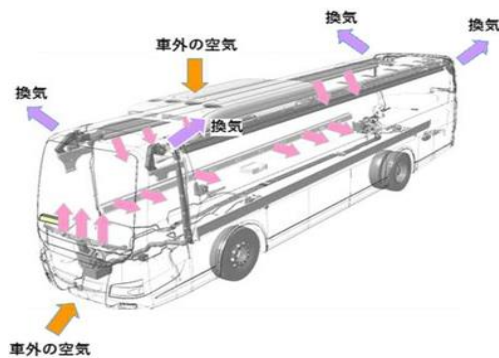
大型観光バス・天井A/Cタイプ
