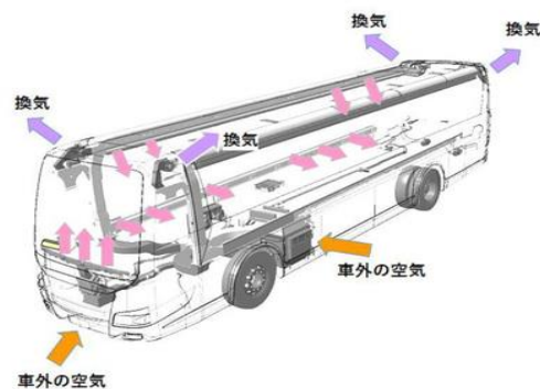
大型観光バス・床下A/Cタイプ
